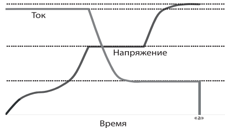
Рис. 3 Зависимость тока и напряжения заряда от времени в режиме IU1, включая фазу заряда малым током и отключение батареи от зарядного устройства (IU1a).
